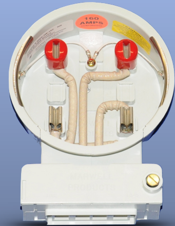
2000-3W-160-NR SHOWN
